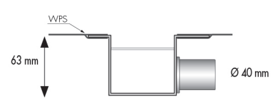
1 | Duschrinnen-Rohbauset 30
