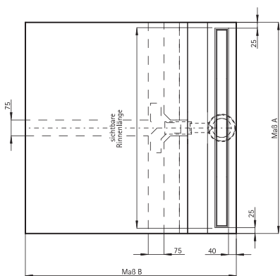
Allgemeine Draufsicht
