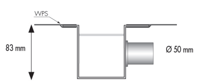
2 | Duschrinnen-Rohbauset 50
