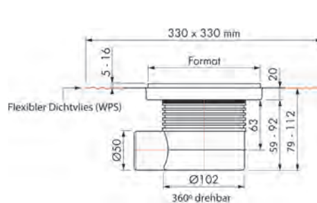
Design Punktabläufe Aqua Jewels waagrecht
