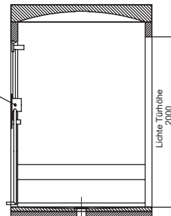
Seitenansicht Schnitt B-B
