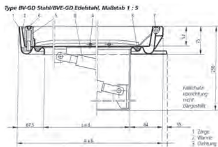
Maßansicht Schachtabdeckung – Typ BV-GD Stahl und BVE-GD Edelstahl
