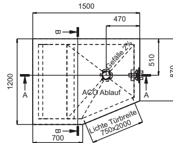
Draufsicht
