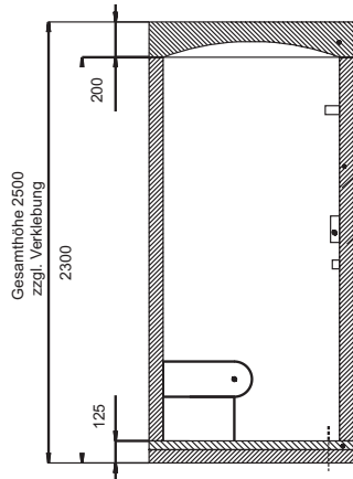
Ansicht von vorn Schnitt A-A
