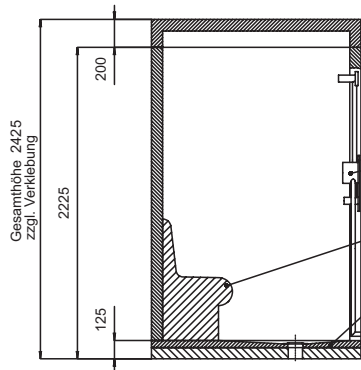
Ansicht von vorn Schnitt A-A
