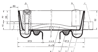
Maßansicht Schachtabdeckung – Typ BVE 33 Edelstahl
