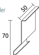
Außenecke 90°
