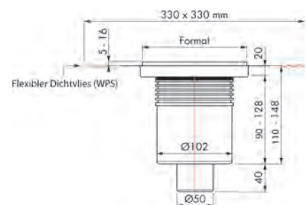
Design Punktabläufe Aqua Jewels senkrecht
