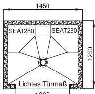
Draufsicht ohne Decke
