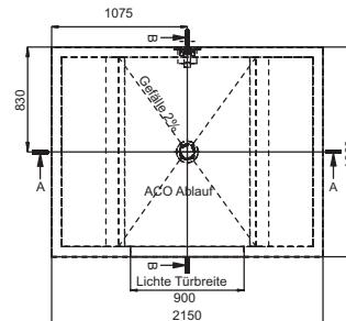
Draufsicht
