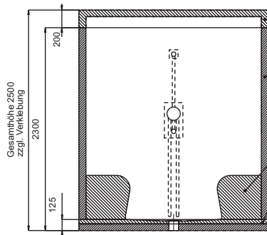
Ansicht von vorn Schnitt A-A
