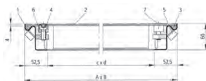
Maßansicht Schachtabdeckung – Typ RV Stahl
