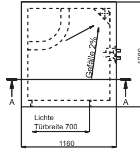
Draufsicht
