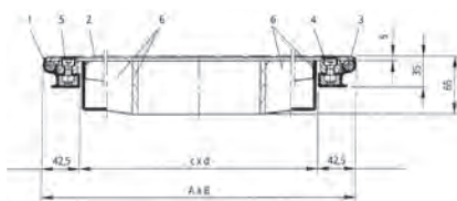
Maßansicht Schachtabdeckung – Typ RVA Aluminium
