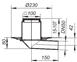
Balkonablauf waagrecht
