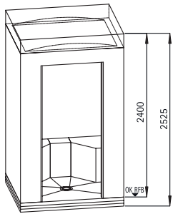
Dimetrische Ansicht
