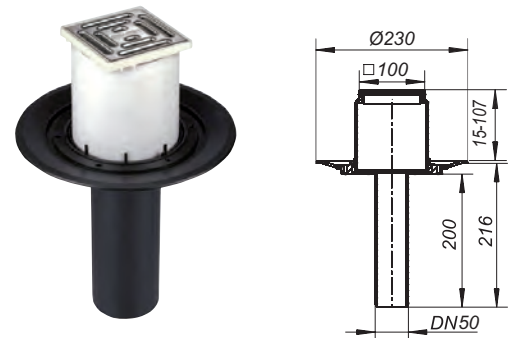
Balkonablauf senkrecht
