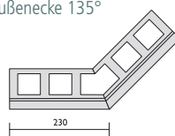
Außenecke 135°
